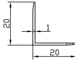
FC-10284 0.100 kg/m
