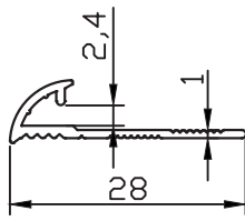
PR-10107 0.108 kg/m
