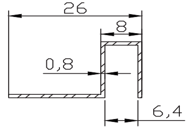
FC-5233 0.111 kg/m
