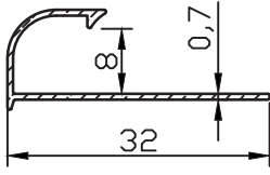
FC-9888 0.103 kg/m
