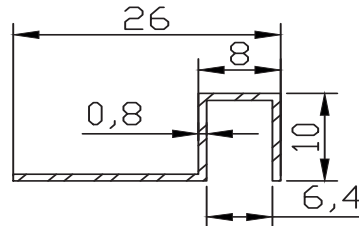
FC-5232 0.100 kg/m
