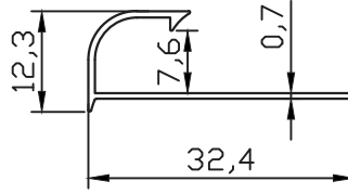
FC-5099 0.108 kg/m
