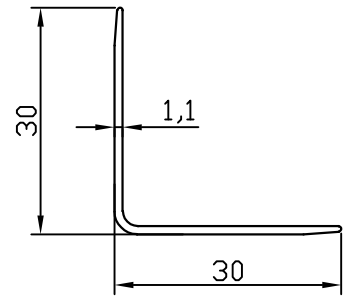
FC-10148 0.168 kg/m
