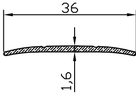
PR-10371 0.133 kg/m
