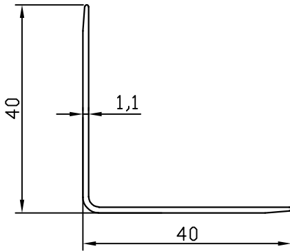
FC-10153 0.228 kg/m
