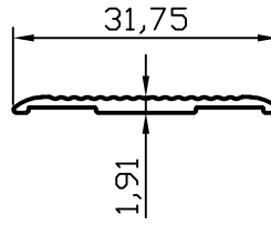
PR-10306 0.119 kg/m
