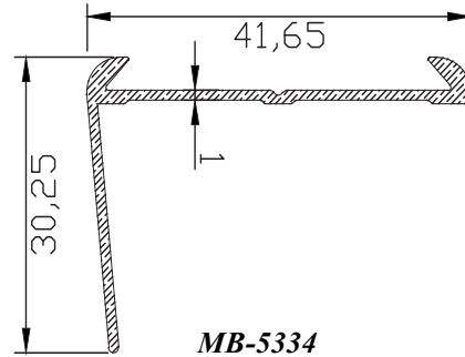
MB-5334 0.171 kg/m
