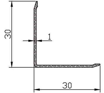
FC-10426 0.157 kg/m
