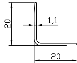
FC-10147 0.108 kg/m
