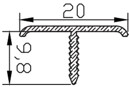
PR-10134 0.092 kg/m
