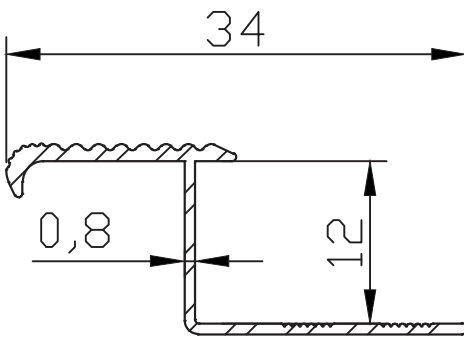
MB-10132 0.125 kg/m
