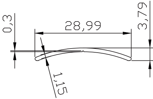
PR-5164 0.092 kg/m
