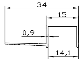
FC-10012 0.144 kg/m
