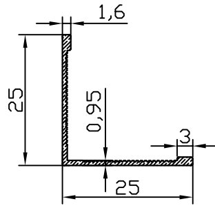
FC-10558 0.125 kg/m
