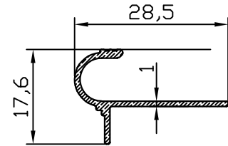
MB-10403 0.141 kg/m
