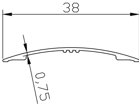
PR-10091 0.098 kg/m
