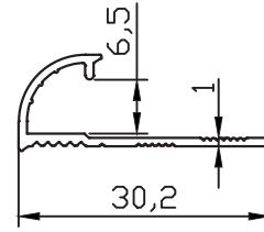
PR-10109 0.133 kg/m
