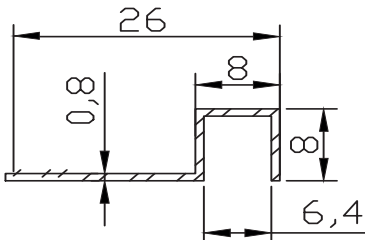
FC-5231 0.092 kg/m
