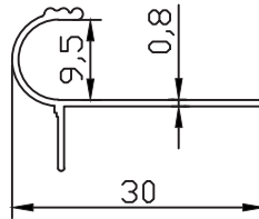
MB-5064 0.111 kg/m
