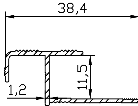
MB-5343 0.195 kg/m
