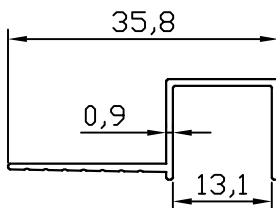
FC-10165 0.146 kg/m
