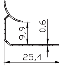
FC-5066 0.084 kg/m
