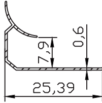
FC-5347 0.079 kg/m
