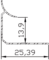
FC-5306 0.089 kg/m
