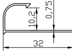
FC-9887 0.113 kg/m
