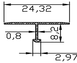
PR-10414 0.073 kg/m
