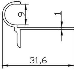
MB-5028 0.154 kg/m
