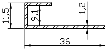
PR-9089 0.185 kg/m
