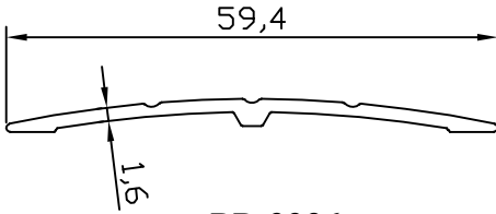
PR-9986 0.266 kg/m
