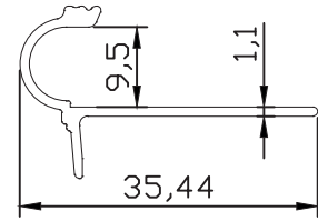
MB-10126 0.189 kg/m
