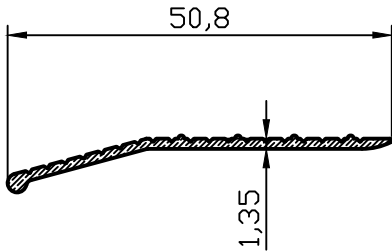
PR-10309 0.184 kg/m
