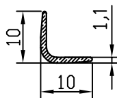
FC-10420 0.049kg/m
