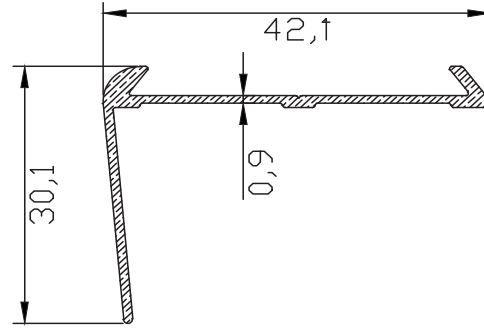
MB-5359 0.228 kg/m
