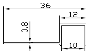
FC-5324 0.141 kg/m
