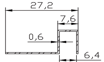
FC-5221 0.076 kg/m
