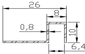
FC-5232 0.100 kg/m
