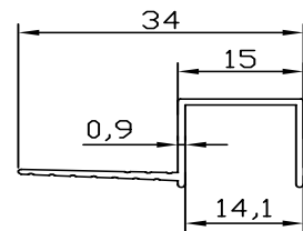
FC-10012 0.144 kg/m
