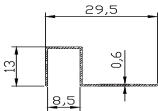
FC-10340 0.088 kg/m
