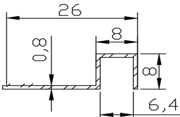
FC-5231 0.092 kg/m
