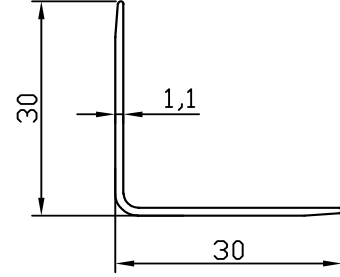
FC-10148 0.168 kg/m
