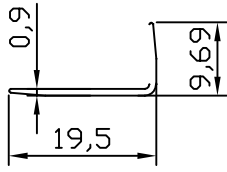
MB-10004 0.062 kg/m
