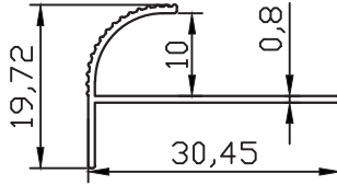
MB-5067 0.124 kg/m
