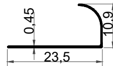
KF-1086 0,046 kg/m
