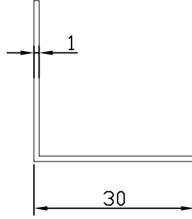
FC-1505 0.160 kg/m
