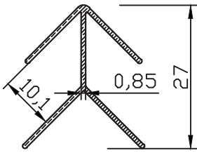
FC-10033 0.176 kg/m
