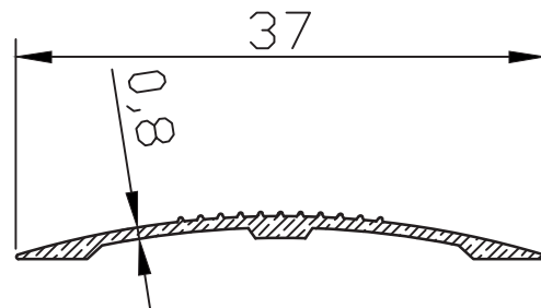
PR-9757 0.097 kg/m
