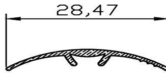
PR-9193 0.102 kg/m
