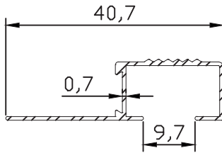
MB-5001 0.150 kg/m
