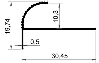
KF-1026 0,081 kg/m
