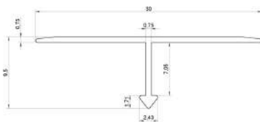
PR-10024 0,081 kg/m
