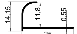
KF-1063 0,065 kg/m
