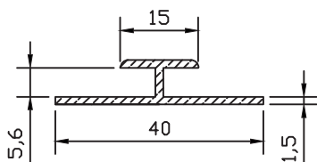
PR-9398-A 0.255 kg/m
