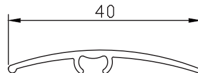
PR-5190 0.166 kg/m
