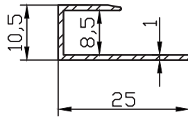
PR-9212 0.122 kg/m
