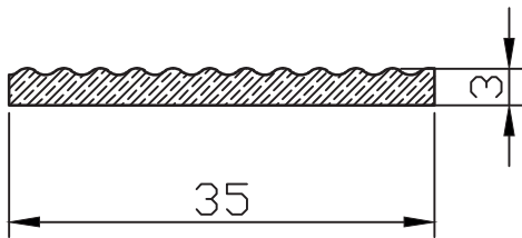
PR-9031 0.260 kg/m
