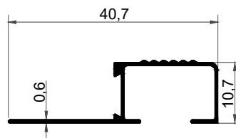
KF-1023 0,130 kg/m
