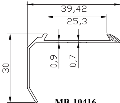
MB-10416 0.195kg/m
