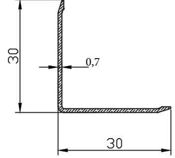
FC-10426 0.114kg/m
