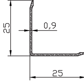
FC-10425 0.119 kg/m
