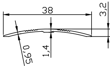
PR-5058 0.095 kg/m
