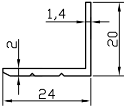
MB-9050 0.192 kg/m
