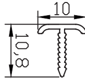
PR-10133 0.065 kg/m
