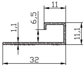
FC-10443 0.147 kg/m
