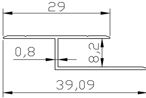
PR-9553 0.132 kg/m
