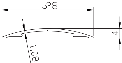
PR-5179 0.121 kg/m
