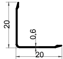
KF-10487 0,070 kg/m
