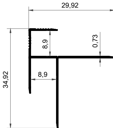
KF-1035 0,163 kg/m
