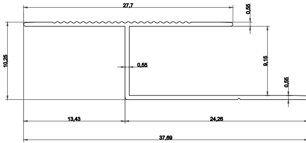
PR-95531 0.122 kg/m
