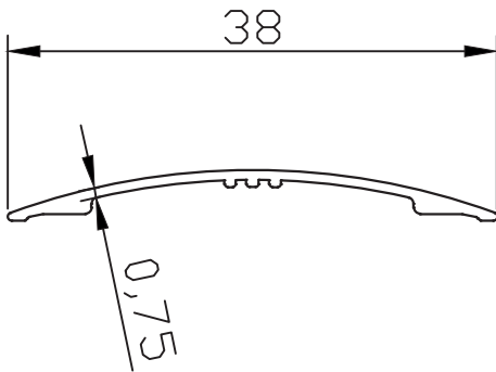
PR-10091 0.098 kg/m
