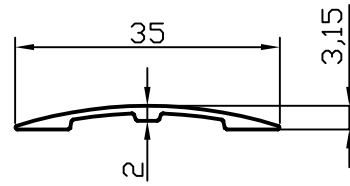
PR-5004 0.119 kg/m
