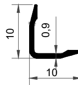
KF-1021 0,043 kg/m
