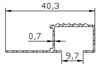
MB-5352 0.157 kg/m
