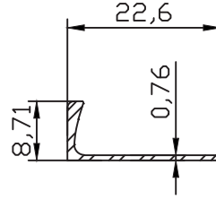
FC-5072 0.079 kg/m
