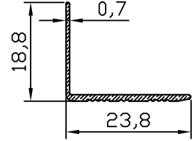
MB-10398 0.103 kg/m
