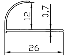
FC - 10014 0.087 kg/m
