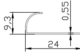
FC-10216 0.054 kg/m
