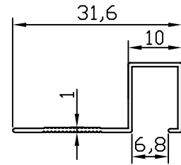
FC-10268 0.117 kg/m
