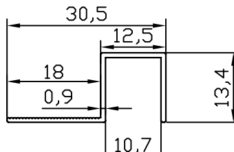
FC-10421 0.133 kg/m
