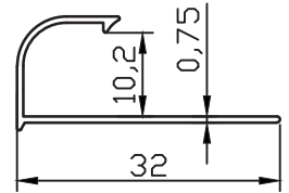
FC-9887 0.113 kg/m
