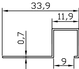
FC-10269 0.114 kg/m
