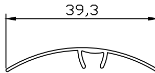
PR-5184 0.105 kg/m
