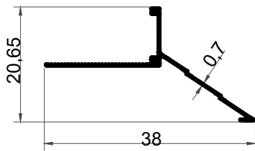
KF-1076 0,114 kg/m
