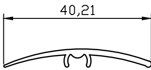
PR-9192 0.174 kg/m
