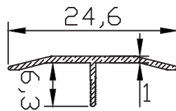
PR-10023 0,073 kg/m
