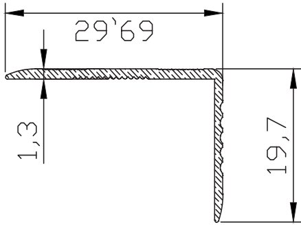
MB-10005 0.144 kg/m
