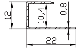
PR-10181 0.095 kg/m
