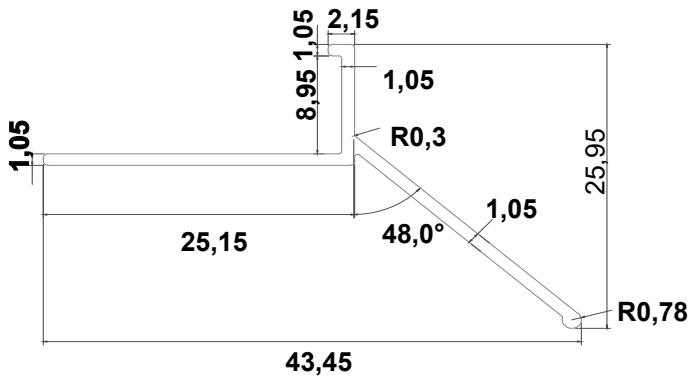
FC-2021 0,174 kg/m
