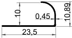
KF-1000 0,046 kg/m
