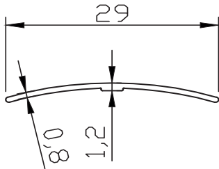
PR-9582 0.067 kg/m
