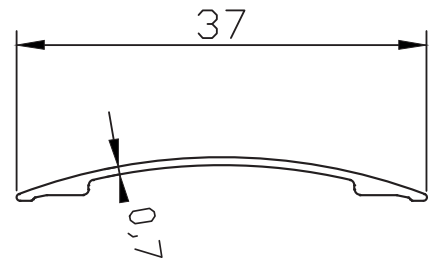
PR-10177 0.089 kg/m
