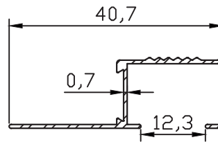
MB-10185 0.152 kg/m
