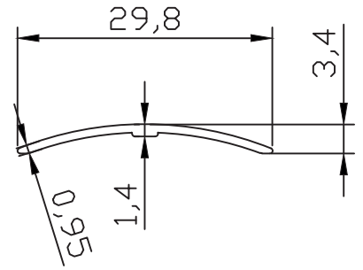
PR-5074A 0.076 kg/m
