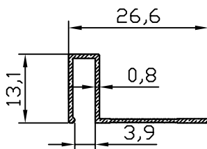
FC-10384 0.109 kg/m
