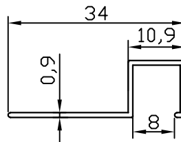
FC-10199 0.133 kg/m
