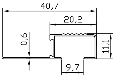
MB-10552 0.130 kg/m
