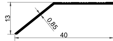
KF-1082 0,098 kg/m
