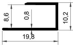
KF-1037 0,087 kg/m
