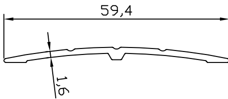
PR-9986 0.266 kg/m
