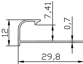
FC-5002 0.096 kg/m
