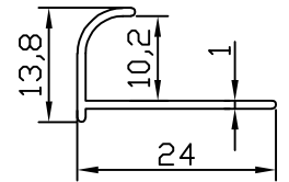
FC - 5341 0.108 kg/m
