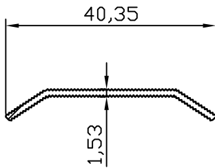
PR-9569 0.139 kg/m
