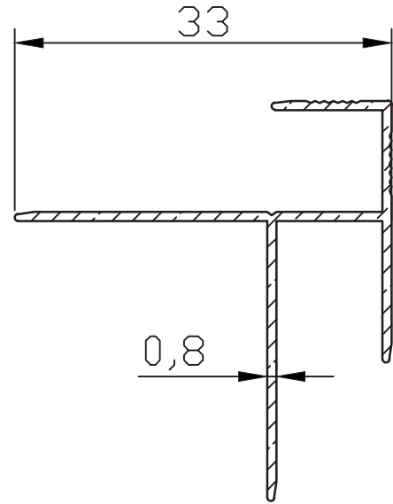
MB-9557 0.187 kg/m
