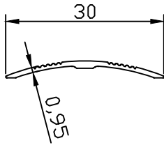
PR-5057 0.076 kg/m
