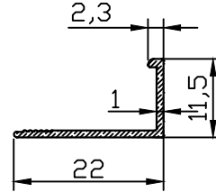
FC-10130 0.089 kg/m
