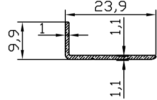
MB-10397 0.092 kg/m
