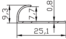
FC-5024 0.081 kg/m
