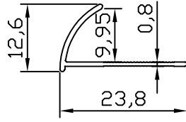
FC-5357 0.084 kg/m
