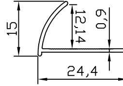
FC-5358 0.100 kg/m
