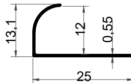
KF-1057 0,062 kg/m
