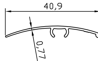
PR-5085 0.124 kg/m
