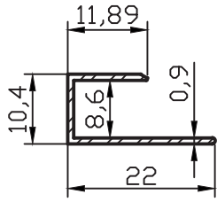
PR-5053 0.103 kg/m
