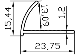
FC-9351 0.125 kg/m
