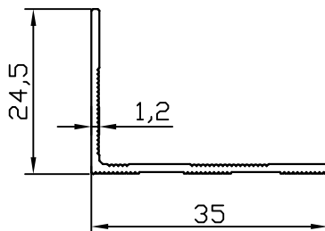
MB-10417 0.184kg/m
