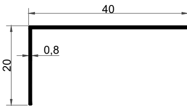
KF-1031 0,127 kg/m
