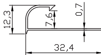
FC-5099 0.108 kg/m
