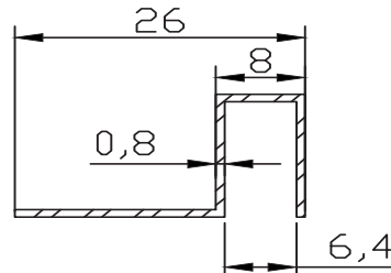
FC-5233 0.111 kg/m
