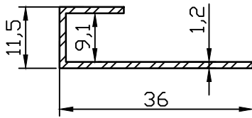
PR-9089 0.185 kg/m
