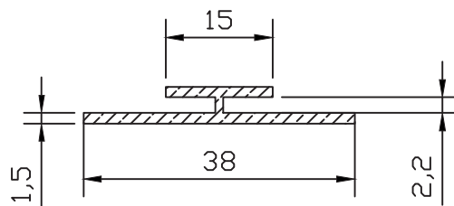
PR-9423 0.222 kg/m
