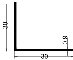
KF-1074 0,144 kg/m
