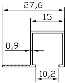
FC-10078 0.146 kg/m
