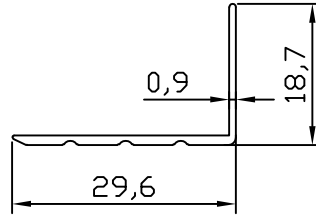
MB-10003 0.138 kg/m
