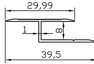
PR-9188 0.152 kg/m
