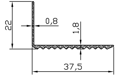
MB-10512 0.173kg/m
