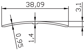
PR-5075A 0.095 kg/m
