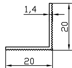
MB-9053 0.119 kg/m
