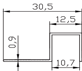
FC-10172 0.133 kg/m
