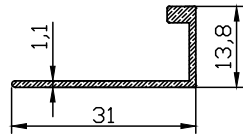
FC-10221 0.157 kg/m
