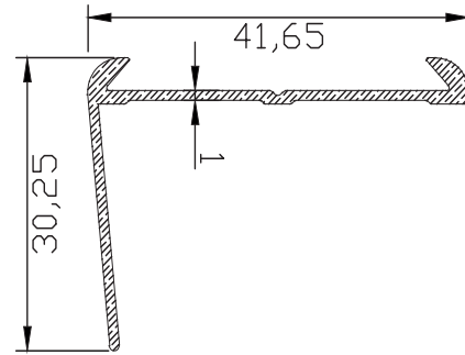
MB-5334 0.171 kg/m
