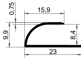
KF-1038 0,087 kg/m
