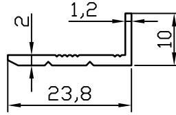
MB-9051 0.148 kg/m
