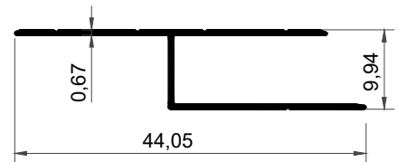
KF-1081 0,130 kg/m
