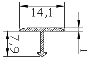
PR-5174 0.062 kg/m
