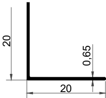
KF-1073 0,070 kg/m
