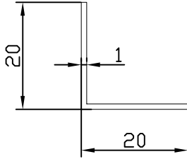
FC-1501 0.106 kg/m
