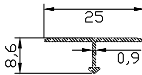
PR-10387 0.082 kg/m
