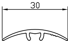
PR-10559 0.127 kg/m
