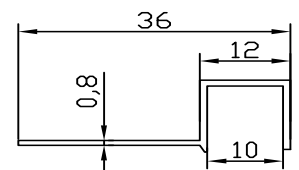
FC-5324 0.141 kg/m
