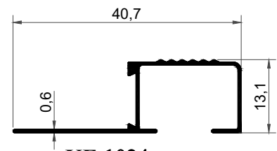
KF-1024 0,136 kg/m
