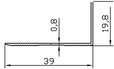
MB-9587 0.134 kg/m
