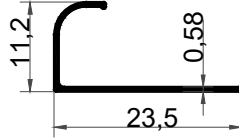
KF-1068 0.060 kg/m
