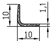
FC-10420 0.049kg/m
