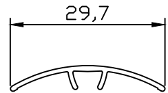
PR-5185 0.092 kg/m
