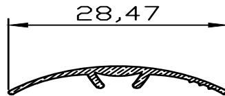
PR-9193 0.102 kg/m
