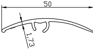
PR-10254 0.257 kg/m
