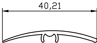
PR-9192 0.174 kg/m
