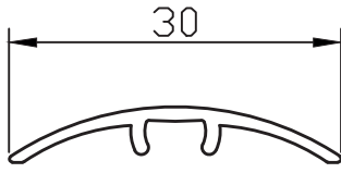
PR-5186 0.115 kg/m
