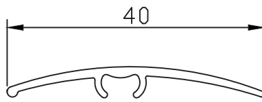
PR-5190 0.166 kg/m
