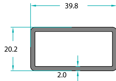
UP-11407 0,152 Kg/m
