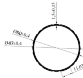
UP-130008 0,584 kg/m
