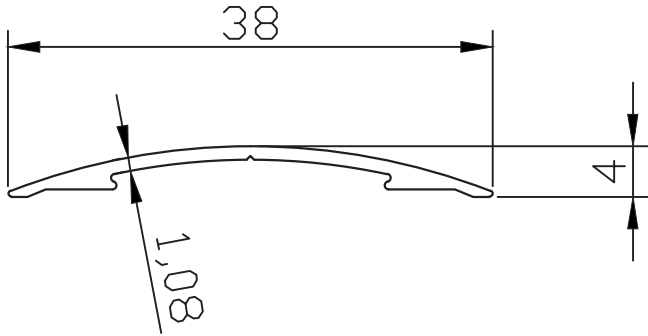
PR-5179 0.121 kg/m
