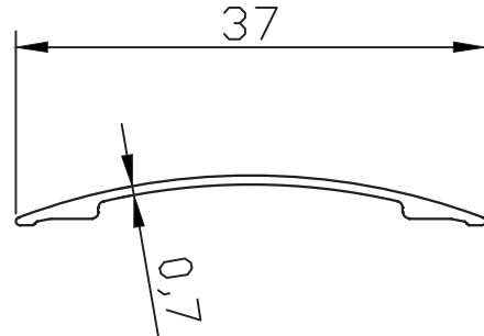
PR-10177 0.089 kg/m
