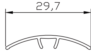
PR-5185 0.092 kg/m
