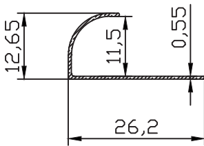
FC-10330 0.068 kg/m
