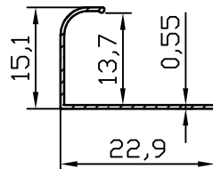
9906 0.063 kg/m
