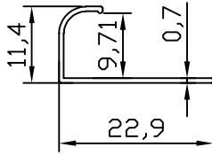
9997 lüks 0.073 kg/m
