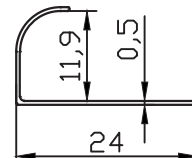
FC-5070 0.054 kg/m
