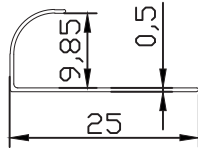
FC-5025 0.050 kg/m
