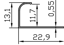
9905 0.060 kg/m
