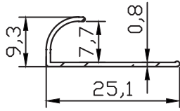
FC-5024 0.081 kg/m
