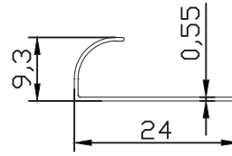
FC-10216 0.054 kg/m
