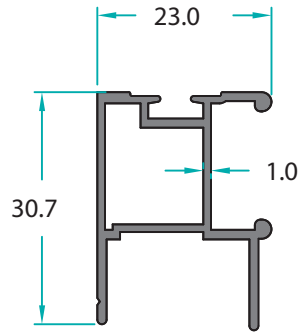
MO-16000 0,344 Kg/m
