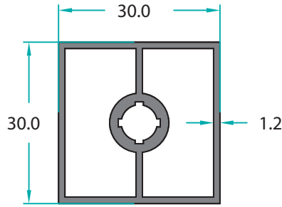
MO-13175 0,764 Kg/m
