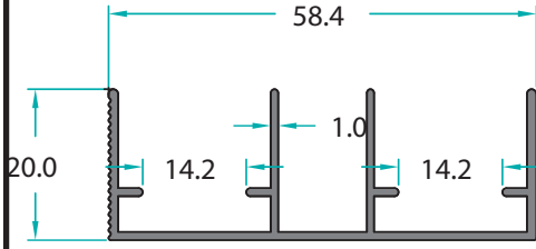
MO-11277 0,439 Kg/m
