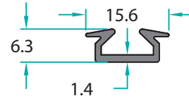
MO-15155 0,100 Kg/m
