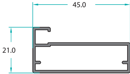
MO-11243 0,434 Kg/m
