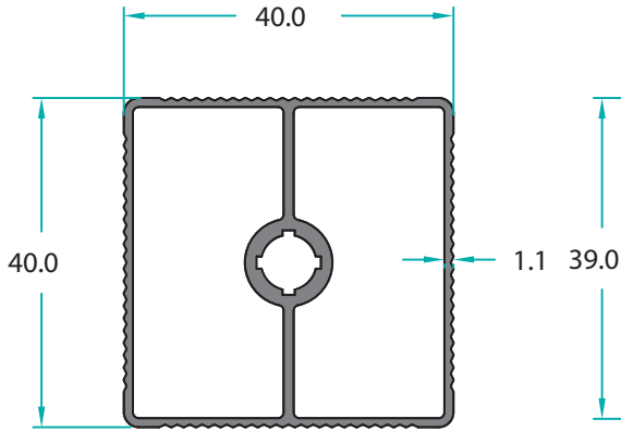
MO-11956 0,631 Kg/m
