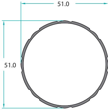
MO-11629 0,545 Kg/m
