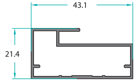
MO-11116 0,396 Kg/m
