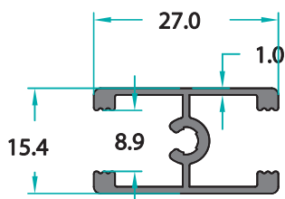
MO-11235 0,287 Kg/m
