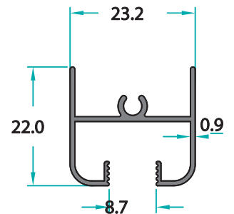
MO-11094 0,222 Kg/m
