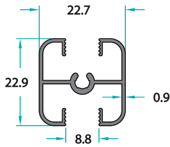
MO-11095 0,266 Kg/m
