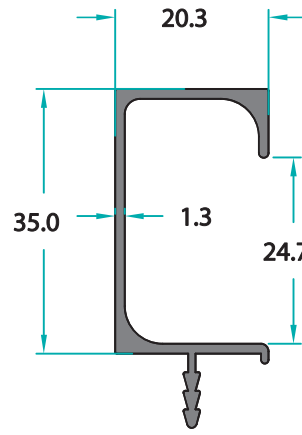
MO-15126 0,358 Kg/m
