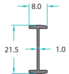
MO-15015 0,111 Kg/m
