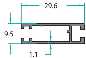
MO-11636 0,234 Kg/m
