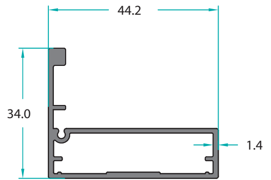
MO-12004 0,531 Kg/m
