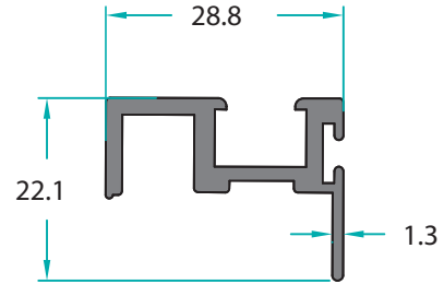
MO-24063 0,401 Kg/m
