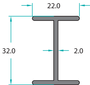
MO-13661 0,388 Kg/m
