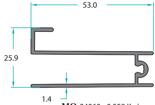
MO-24060 0,558 Kg/m
