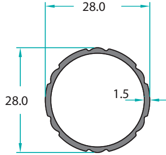
MO-11630 0,314 Kg/m
