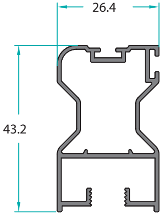
MO-11246 0,518 Kg/m
