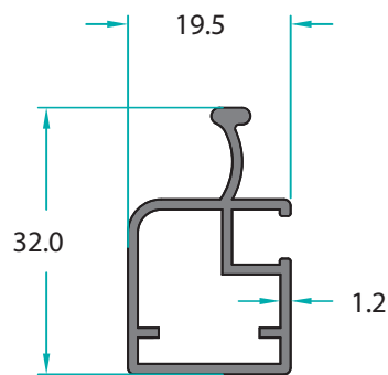
MO-11242 0,347 Kg/m
