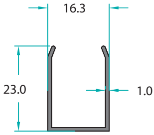
MO-11573 0,165 Kg/m
