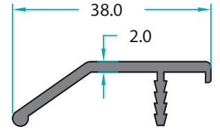
MO-13769 0,282 Kg/m
