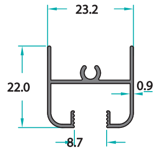
MO-11094 0,222 Kg/m
