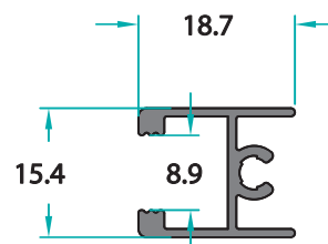
MO-11233 0,209 Kg/m
