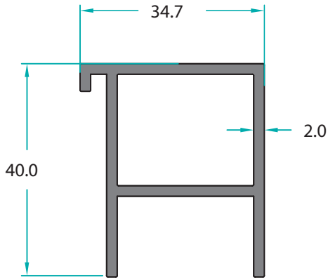
MO-11254 0,759 Kg/m
