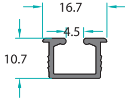
MO-24061 0,144 Kg/m
