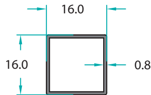
MO-15120 0,133 Kg/m
