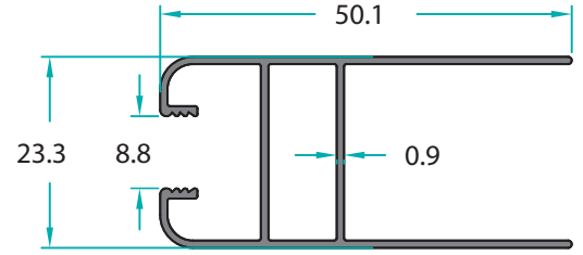
MO-11097 0,393 Kg/m
