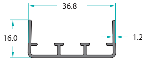
MO-7490 0,271 Kg/m
