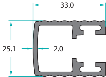
MO-11567 0,612 Kg/m
