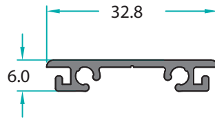
MO-11378 0,220 Kg/m
