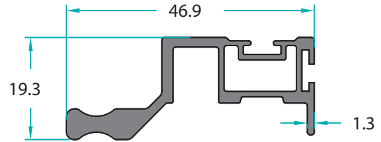
MO-11230 0,564 Kg/m
