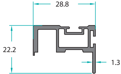
MO-11229 0,371 Kg/m
