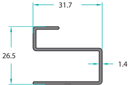
MO-11228 0,331 Kg/m
