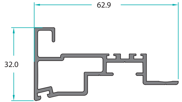
MO-15017 0,732 Kg/m
