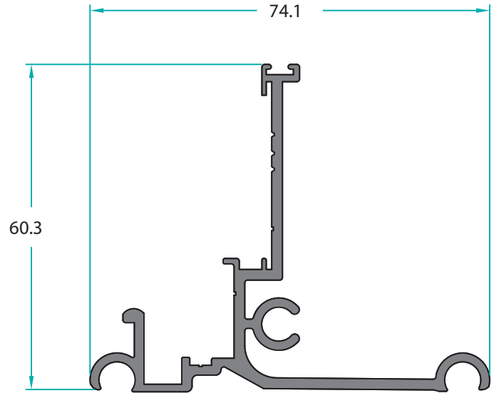
MO-13471 0,279 Kg/m
