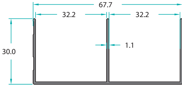
MO-11258 0,453 Kg/m
