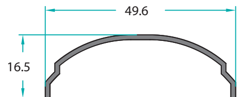
MO-11474 0,225 Kg/m
