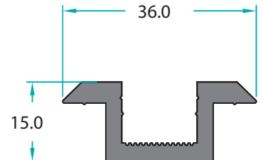
MO-13712 0,509 Kg/m
