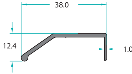
MO-16005 0,225 Kg/m
