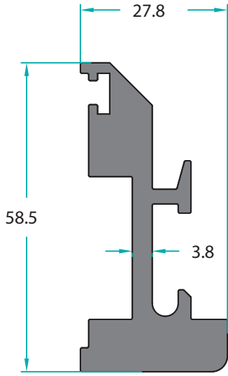
MO-11328 1,696 Kg/m
