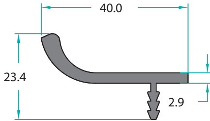
MO-11263 0,442 Kg/m
