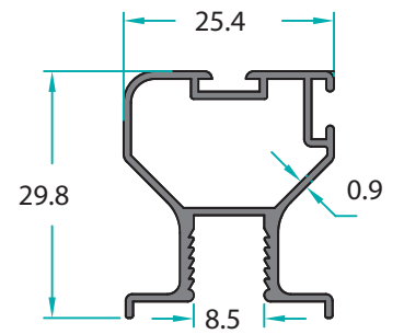
MO-11096 0,341 Kg/m
