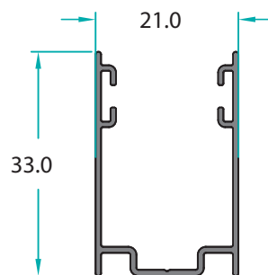
MO-13698 0,238 Kg/m
