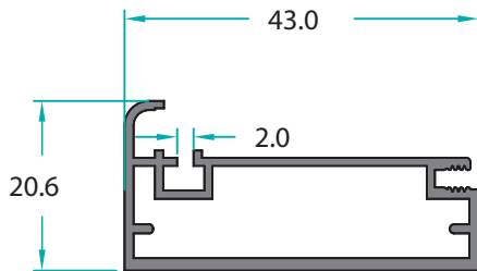
MO-11369 0,455 Kg/m
