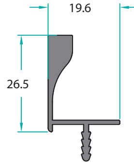
MO-15124 0,347 Kg/m
