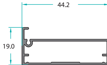
MO-12003 0,374 Kg/m
