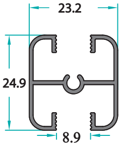
MO-11255 0,301 Kg/m
