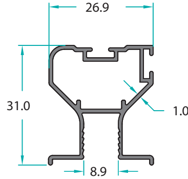
MO-11309 0,355 Kg/m
