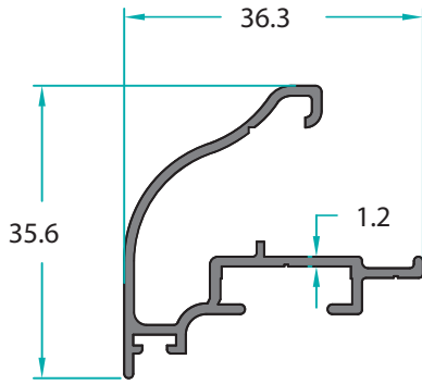
MO-13340 0,369 Kg/m
