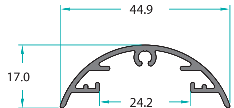
MO-11381 0,331 Kg/m
