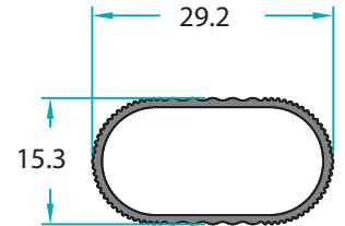
MO-11271 0,195 Kg/m
