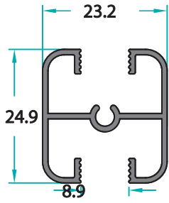
MO-11255 0,301 Kg/m
