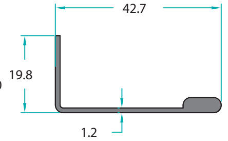
MO-11239 0,420 Kg/m
