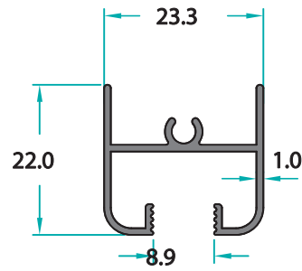
MO-11256 0,244 Kg/m
