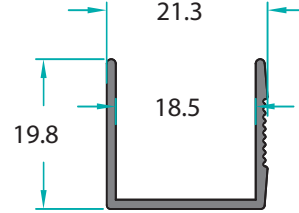
MO-11274 0,192 Kg/m
