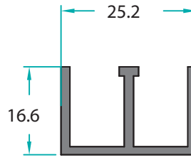
MO-13112 0,320 Kg/m
