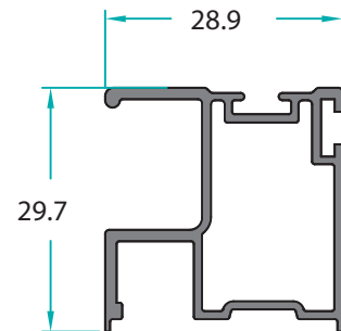
MO-11231 0,420 Kg/m
