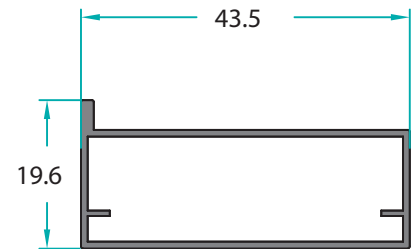
MO-11098 0,312 Kg/m
