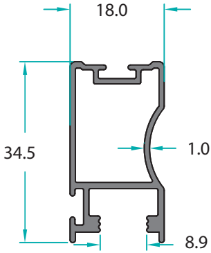
MO-11236 0,360 Kg/m
