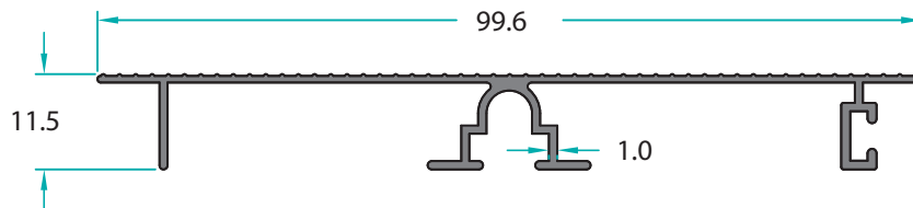
MO-11239 0,421 Kg/m
