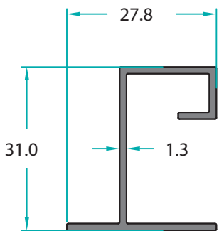
MO-11311 0,314 Kg/m
