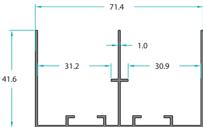
MO-15128 0,618 Kg/m
