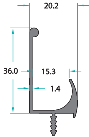
MO-15051 0,369 Kg/m
