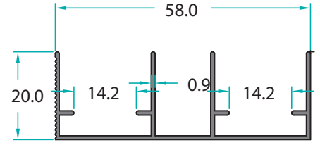
MO-15249 0,355 Kg/m
