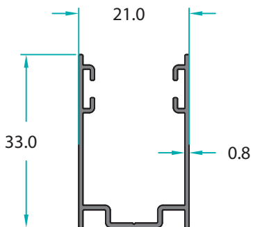
MO-15016 0,241 Kg/m
