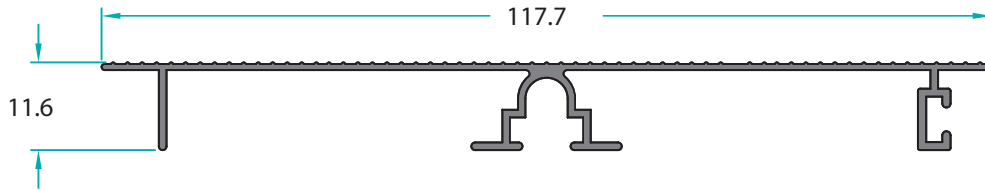
MO-11238 0,469 Kg/m
