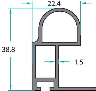
MO-11297 0,577 Kg/m
