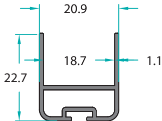
MO-11275 0,263 Kg/m
