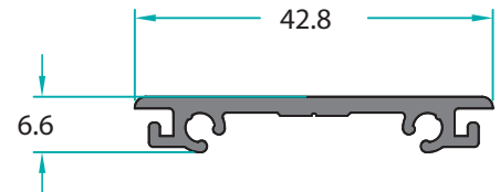
MO-11382 0,322 Kg/m
