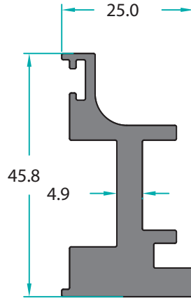
MO-11326 1,138 Kg/m
