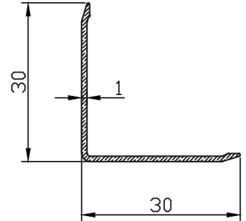
FC-10426 0.157 kg/m
