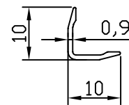
A 10536 0.043kg/m
