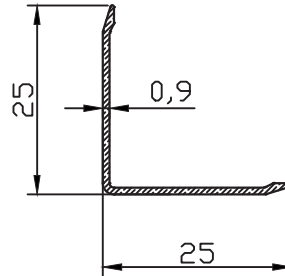
FC-10425 0.119 kg/m
