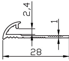
PR-10107 0.108 kg/m
