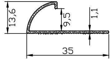
PR-10441 0.152 kg/m
