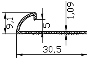
PR-10439 0.121 kg/m
