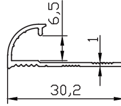
PR-10109 0.133 kg/m
