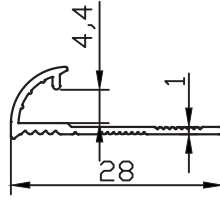
PR-10108 0.114 kg/m
