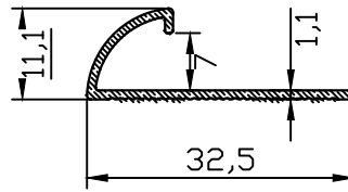
PR-10440 0.134 kg/m
