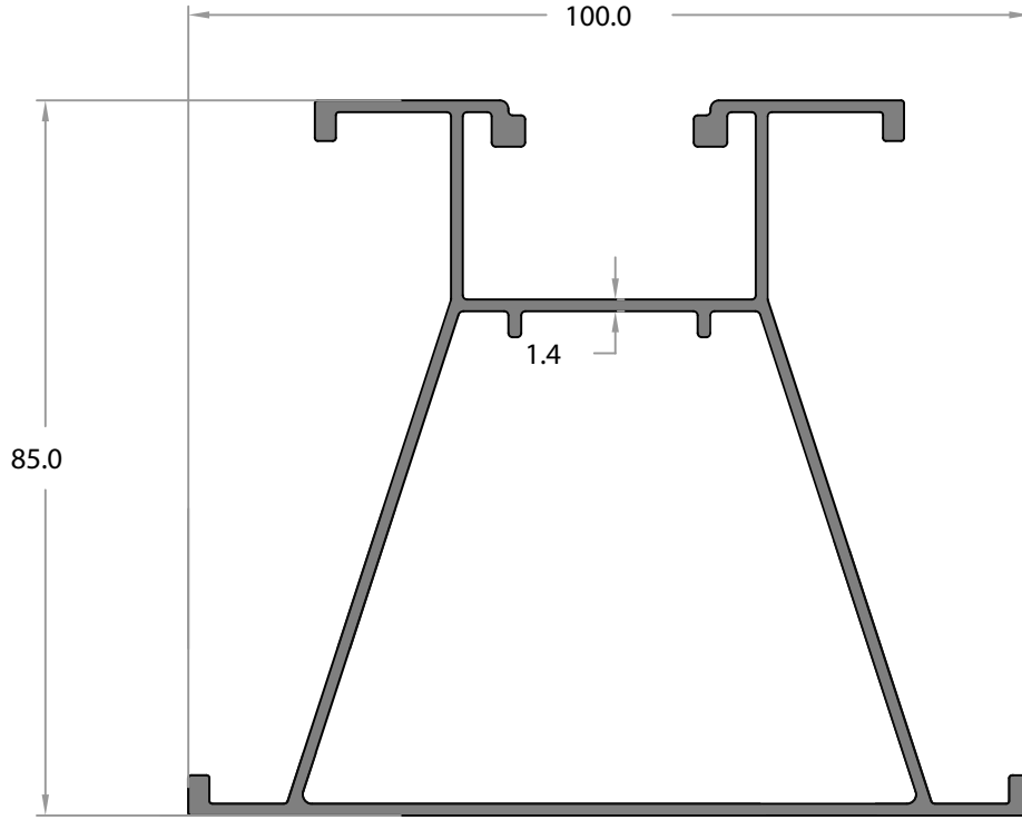
GE-14135 1,539 Kg/m
