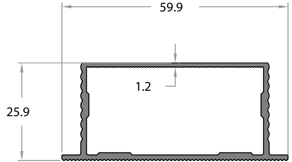
GE-11488 0,588 Kg/m
