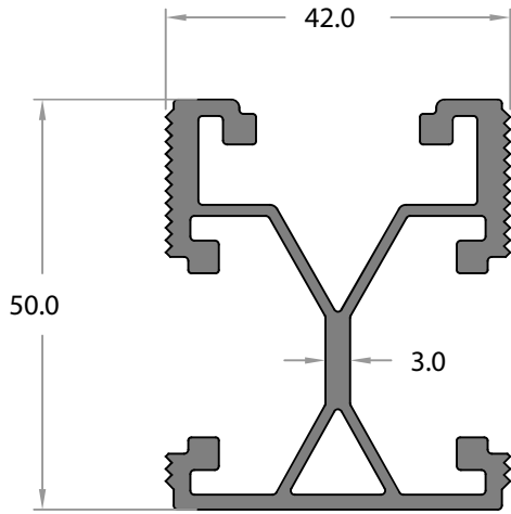
GE-13803 0,713 Kg/m
