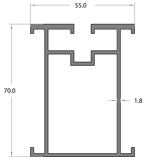
GE-13662 1,558 Kg/m
