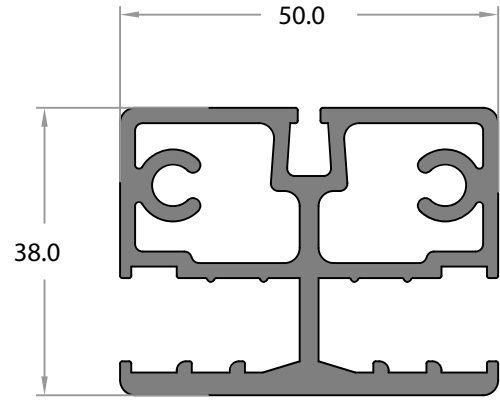
GE-13811 1,718 Kg/m
