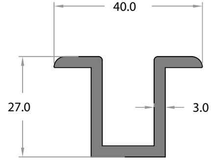
GE-13011 0,705 Kg/m
