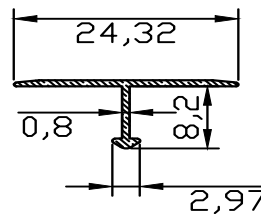
PR-10414 0.073 kg/m
